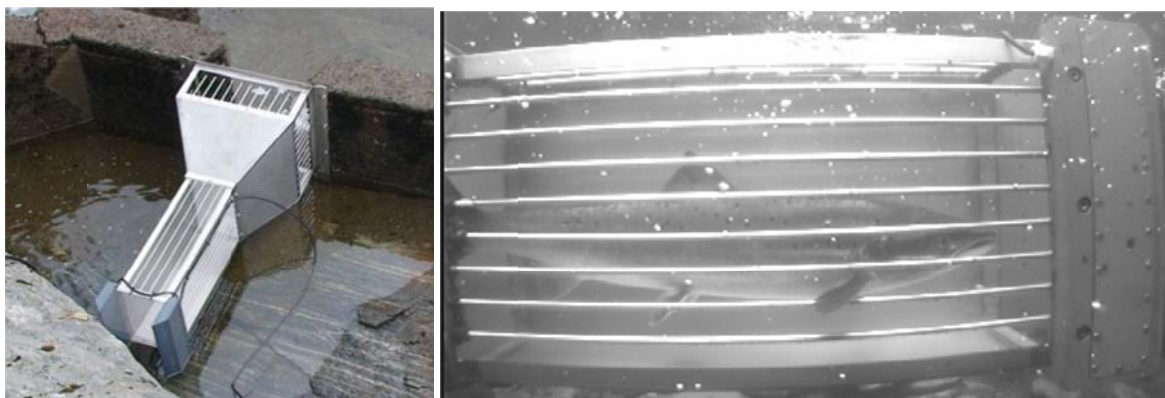
Figur 4 Videoovervåking i fisketrapp. Bildet til venstre viser kalv med målekammer og optisk sensor/utløser. Bildet til høyre viser en villaks inne i målekammeret.
